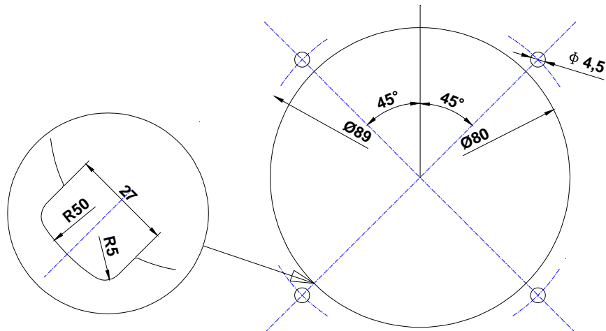
Détail pour instruments avec réglage
