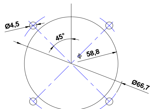
Découpe pour instruments moteur
