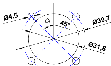
Découpe pour instruments électroniques
